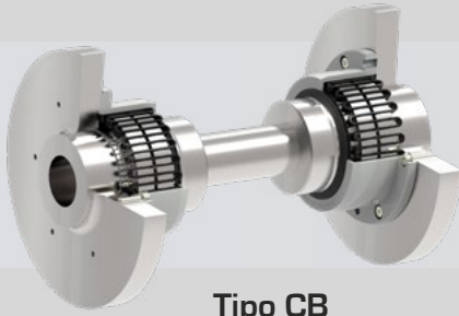
Tipo CB Con eje alargador
